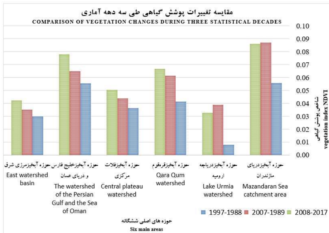
شکل ۲- تغییرات شاخص نرمال‌شده تفاوت پوشش گیاهی (NDVI) در زیرحوضه‌های آبخیز اصلی در سه دوره زمانی ۱۰ ساله Figure 2- Changes of NDVI in main sub-watersheds in three 10-year periods
