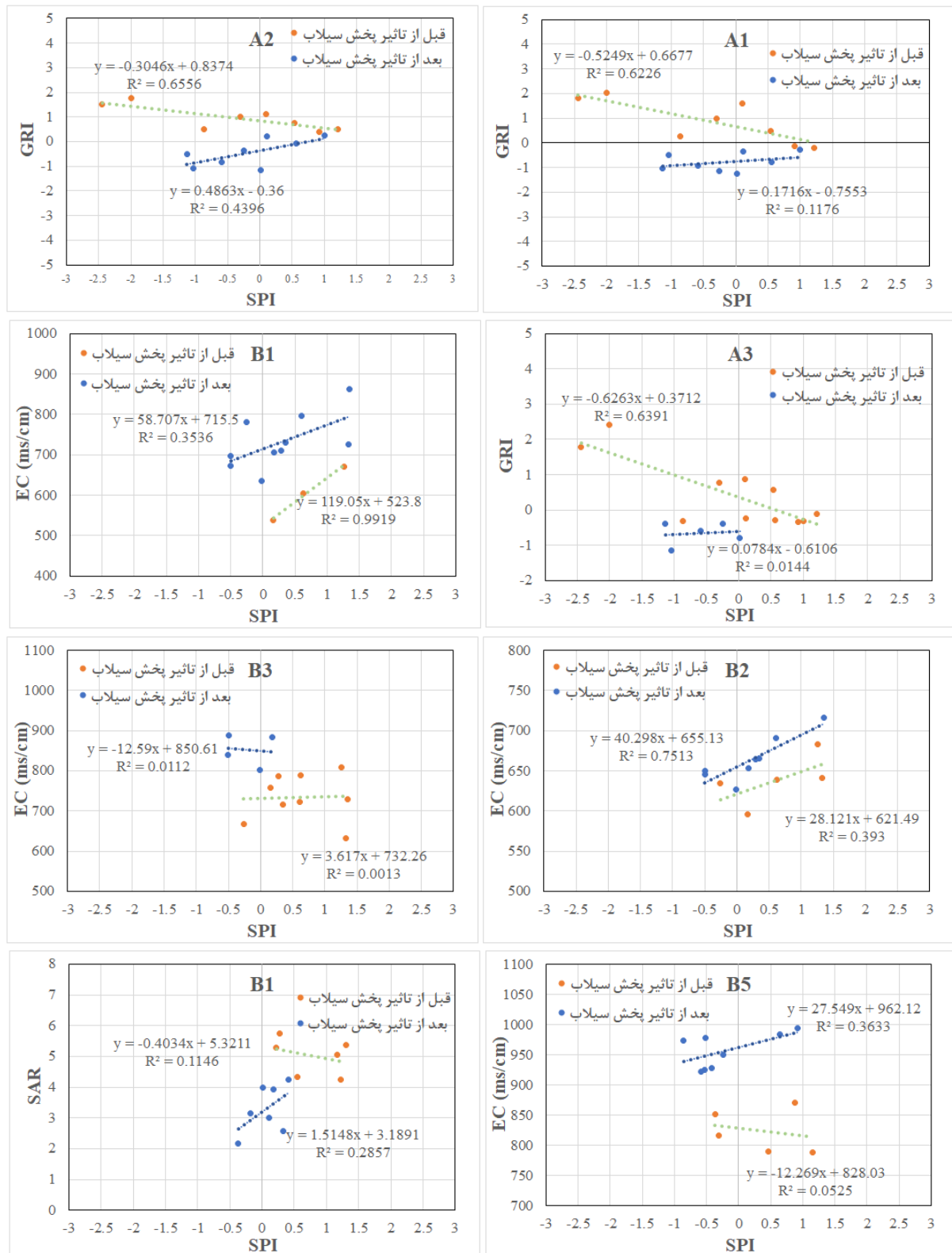
شکل ۷- نمودار اثر پخش سیلاب بر حساسیت شاخص‌های کمی و کیفی چاه‌های انتخابی به خشکسالی
