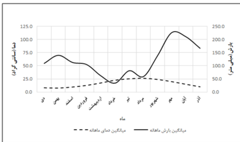
شکل ۳- منحنی آمبروترمیک منطقه مورد مطالعه Figure 3- The ombrothermic diagram of the studied area
