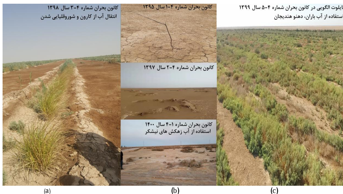
شکل ۳- (a) (b) (c) نمونه‌ای از روش سنتی، پیتینگ و نتایج پایلوت طی چندمرحله مبارزه با ریزگردها
