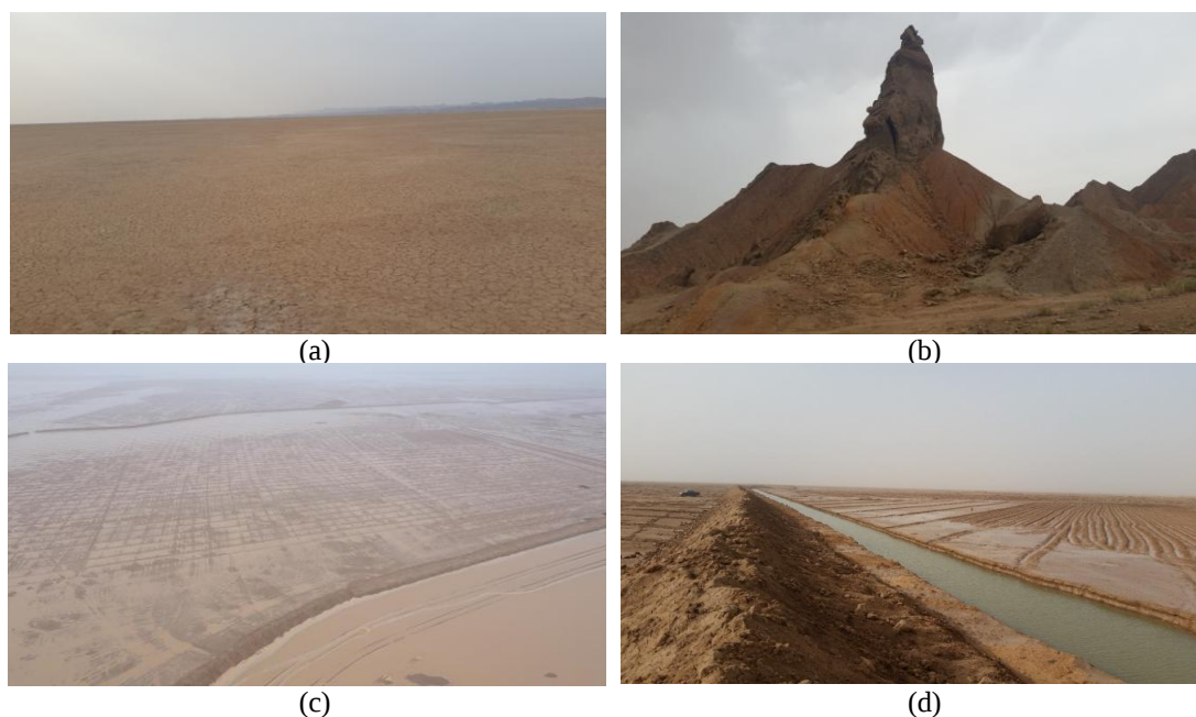
شکل ۲- نمای کلی منطقه انتخابی در سال ۱۳۹۶ (a) (b) قبل از اجرای پژوهش و (c) (d) در سال ۱۳۹۷ پس از اجرای عملیات بیومهندسی، بیولوژیکی، مکانیکی و بیومکانیکی در راستای احیای خاک، زمین و ارتقاء پوشش گیاهی در بافت خاک رسی شور با فرسایش شدید بادی رخنمون در منطقه قابل مشاهده است.
