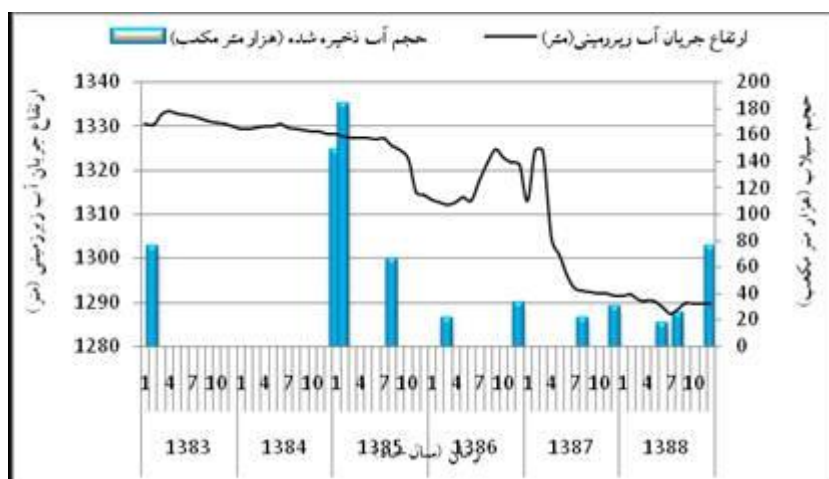
شکل ۹- نمودار تغییرات همزمان ارتفاع جریان آب زیرزمینی و حجم سیلاب ورودی در چاه مشاهده‌ای Pt4
