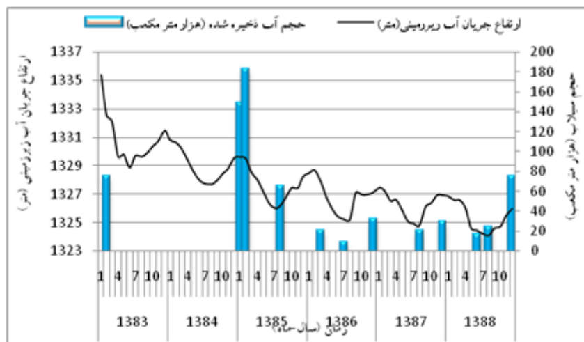
شکل ۸- نمودار تغییرات همزمان ارتفاع جریان آب زیرزمینی و حجم سیلاب ورودی در چاه مشاهده‌ای Pt3
