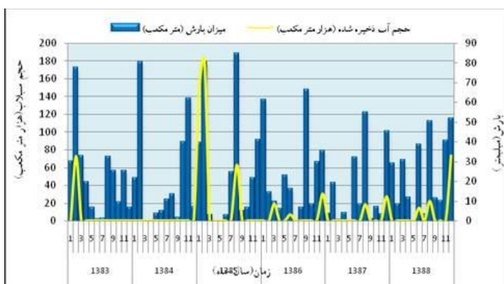
شکل ۵- نمودار تغییرات هم‌زمان بارش و حجم سیلاب ورودی (سال‌های آبی ۸۳-۸۸)
