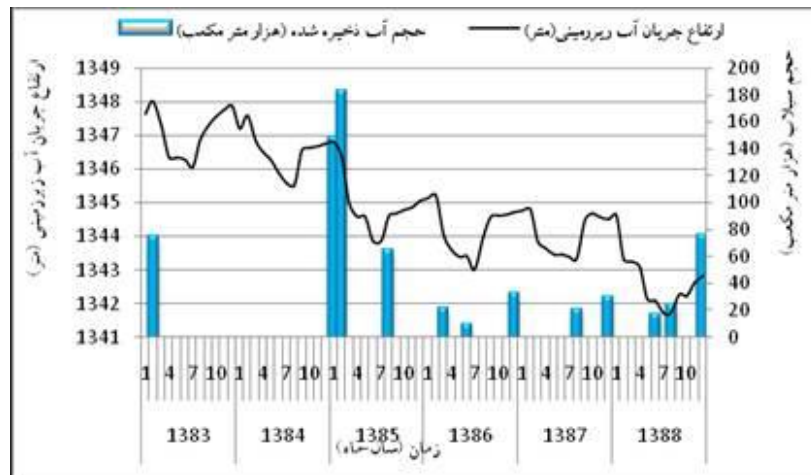
شکل ۷- نمودار تغییرات همزمان ارتفاع جریان آب زیرزمینی و حجم سیلاب ورودی در چاه مشاهده‌ای Pt2
