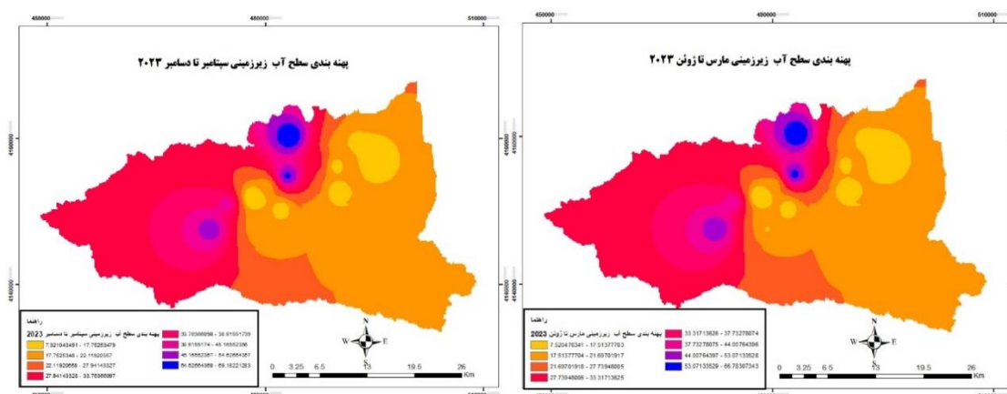
شکل ۵- پهنه‌بندی سطح آب زیرزمینی مارس تا ژوئن ۲۰۲۳ (راست) و سپتامبر تا دسامبر ۲۰۲۳ (چپ) Figure 4- Groundwater level zoning from March to June (Right) and September to December 2023 (Left)
