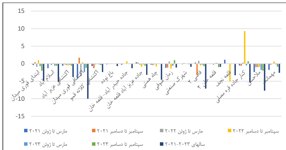
شکل ۱۲- نمودار افت آب زیرزمینی در سری‌های زمانی مختلف
