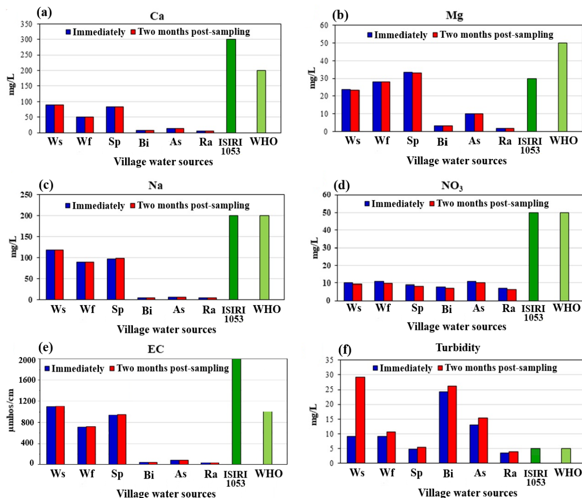
شکل ۲- هیستوگرام مقایسه‌ای پارامترهای فیزیکیوشیمیایی منابع آبی روستای چناران، اندازه‌گیری شده بلافاصله و دو ماه بعد از نمونه‌برداری. باران (Ra)، ایرانیت (As)، ایزوگام (Bi)، چشمه (Sp)، مخزن آب (Ws) و آبشار (Wf)
