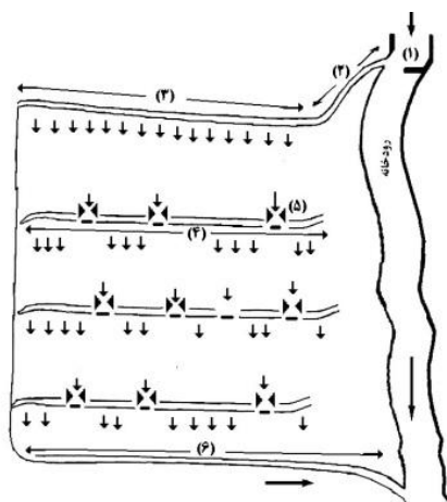
۱- دهانه آبیگیر ۲- نهر آبرسان ۳- نهر آبرسان گسترشی ۴- نهر گسترشی (پخش) ۵- دروازه‌ها ۶- نهر تخلیه آب مازاد شکل ۱- طرح شماتیک یک نوع سامانه پخش سیلاب بر آبخوان به روش مستقیم (اقتباس: وهابی، ۱۳۸۲) Figure 1- Schematic of floodwater spreading system (FWSS) via direct method (Vahabi, 2003)
