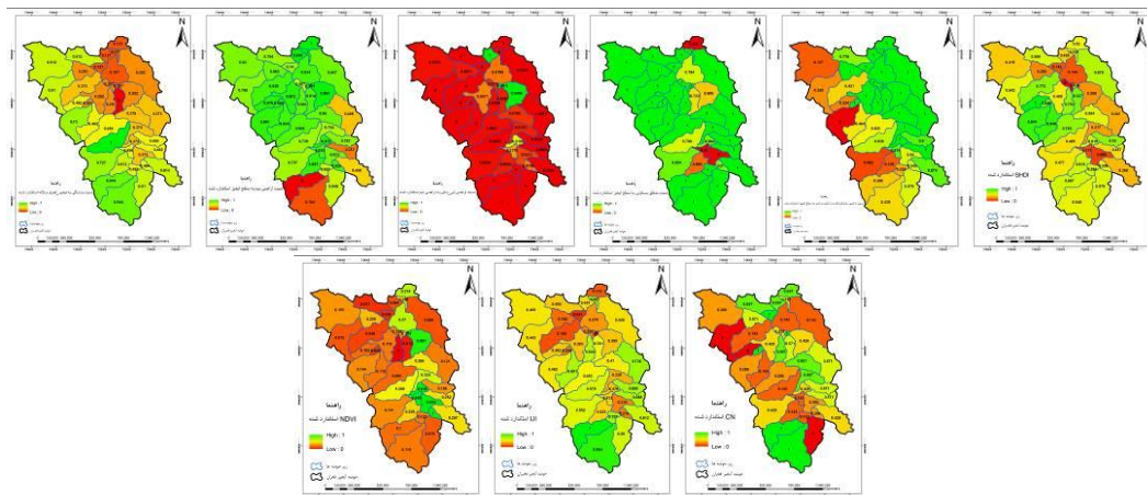
شکل ۶- تغییرات مکانی معیارهای مورد استفاده در شاخص حالت
