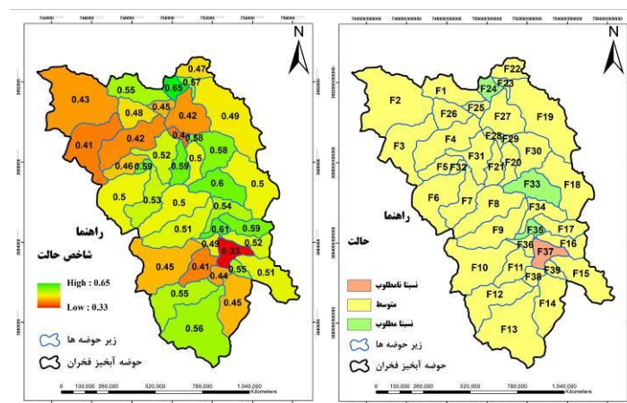
شکل ۷- تغییرات مکانی شاخص حالت در زیرآبخیزهای مختلف
