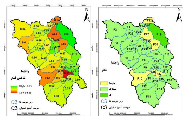
شکل ۵- تغییرات مکانی شاخص فشار در زیر آبخیزهای مختلف
