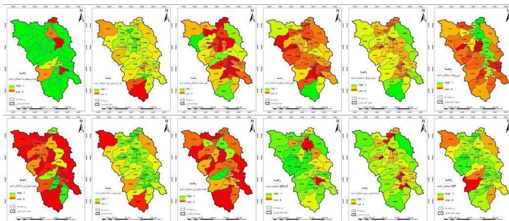
شکل ۸- تغییرات مکانی معیارهای مورد استفاده در شاخص پاسخ
