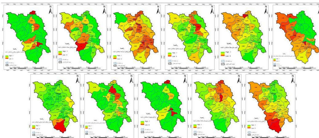
شکل ۴- تغییرات مکانی معیارهای مورد استفاده در شاخص فشار
