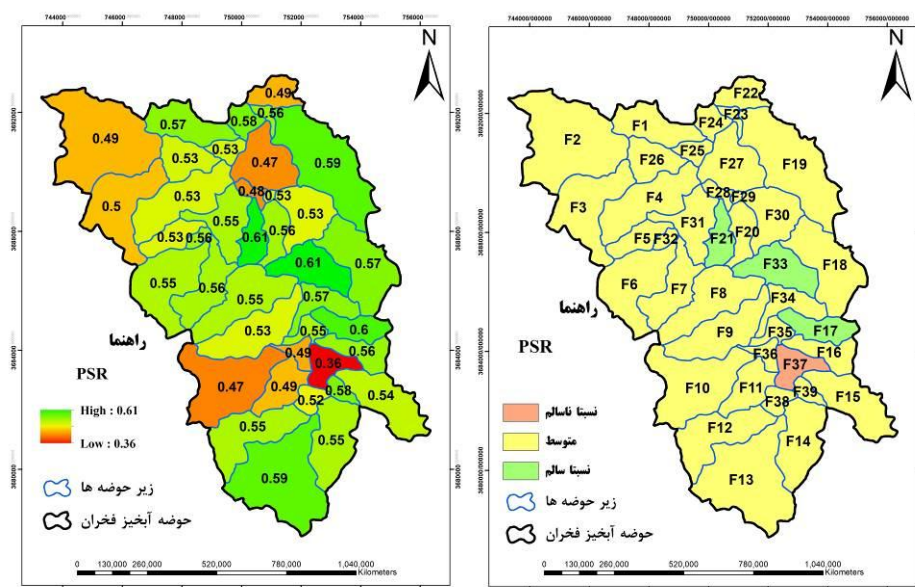
شکل ۱۰- تغییرات مکانی شاخص سلامت در زیرآبگیرهای مختلف
