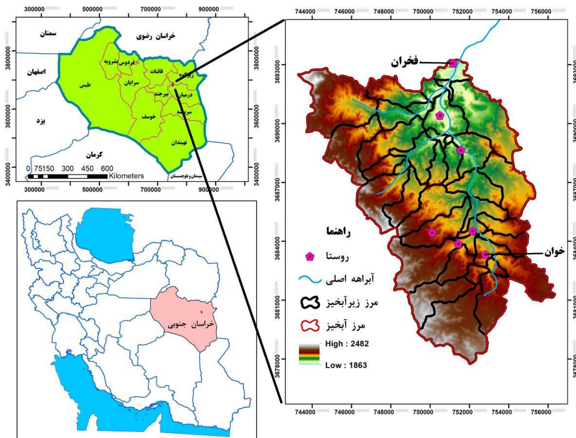
شکل ۱- موقعیت مکانی و پراکنش ارتفاعی آبخیز فخران در خراسان جنوبی و ایران
