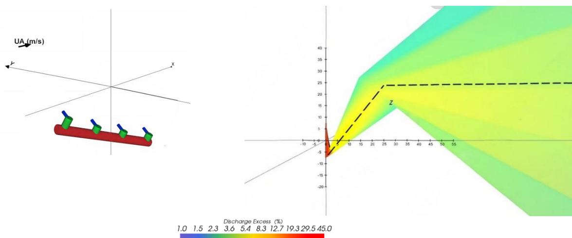
شکل ۳- نمای افقی تغییرات غلظت شوری در مسیر هاله آلودگی
